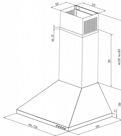
Rys. 1 Rysunek gabarytowy.
