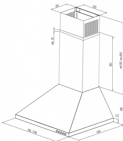
Rys. 1 Rysunek gabarytowy.
