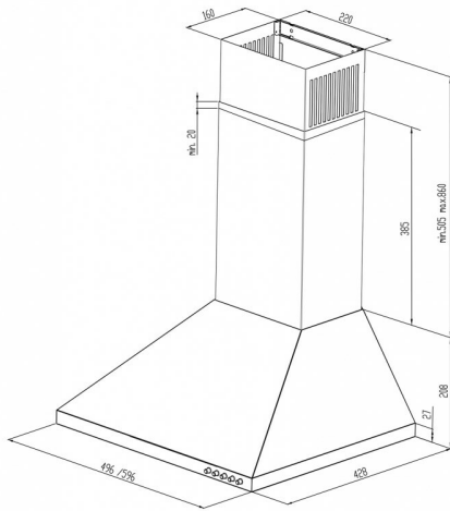
Rys. 1 Rysunek gabarytowy.
