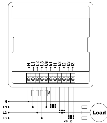
Anschlussdiagramm EM-100D
