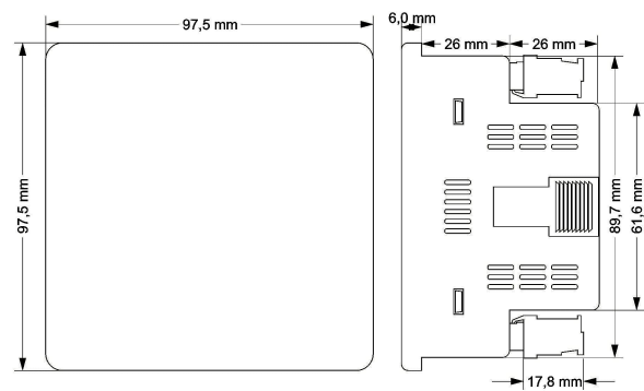
Abmessungen EM-100D
