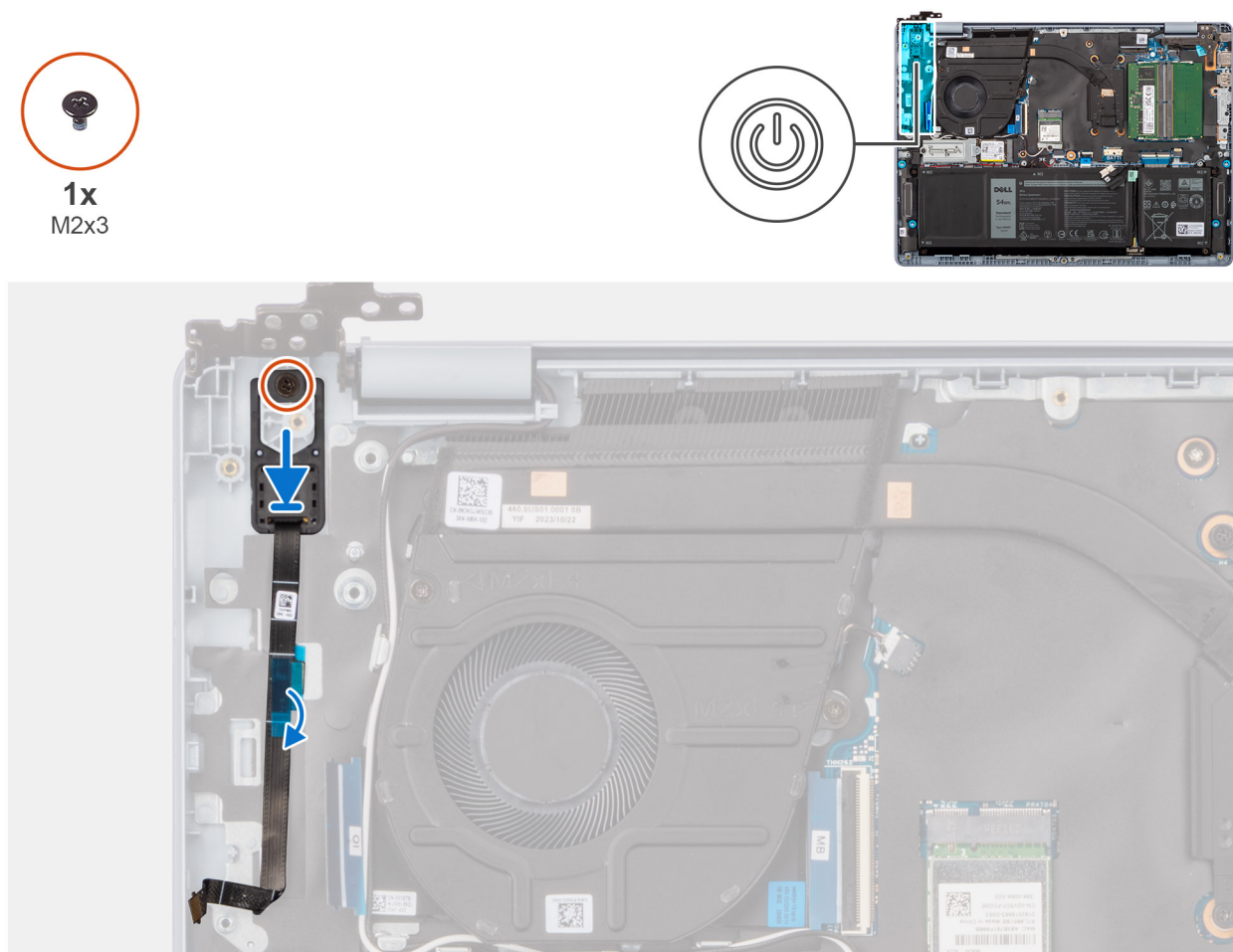
Rysunek 55. Instalowanie przycisku zasilania z czytnikiem linii papilarnych
