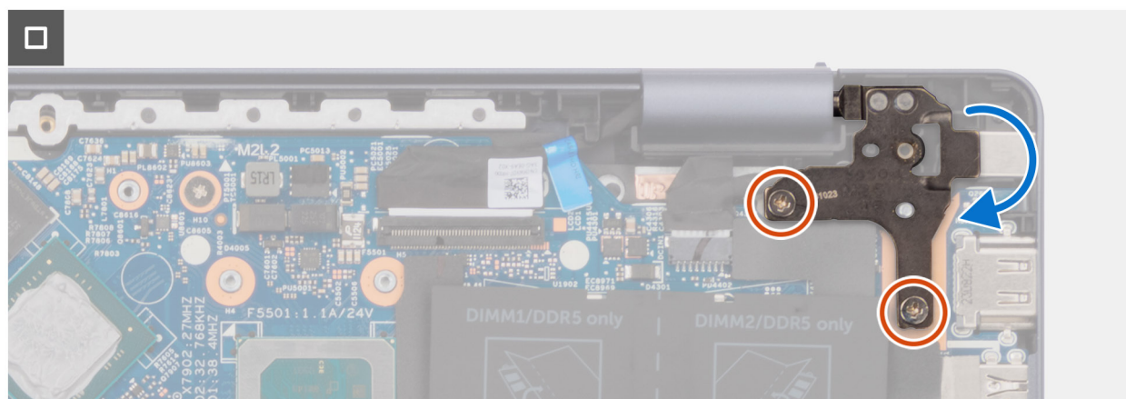
Rysunek 108. Wkręcanie śrub zawiasów
