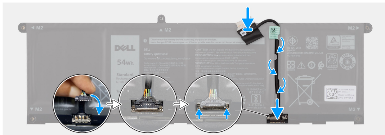
Rysunek 27. Podłączanie kabla baterii
