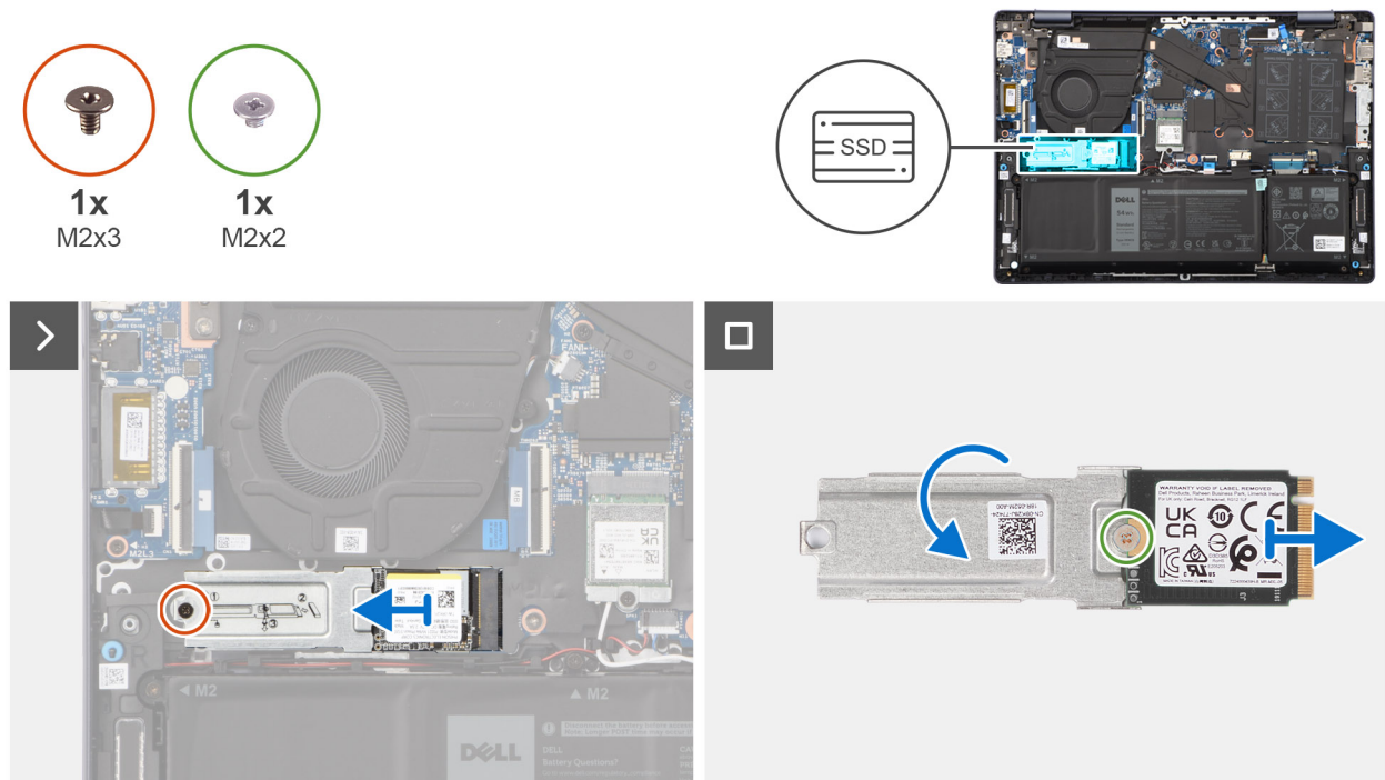
Rysunek 34. Wymontowywanie dysku SSD
