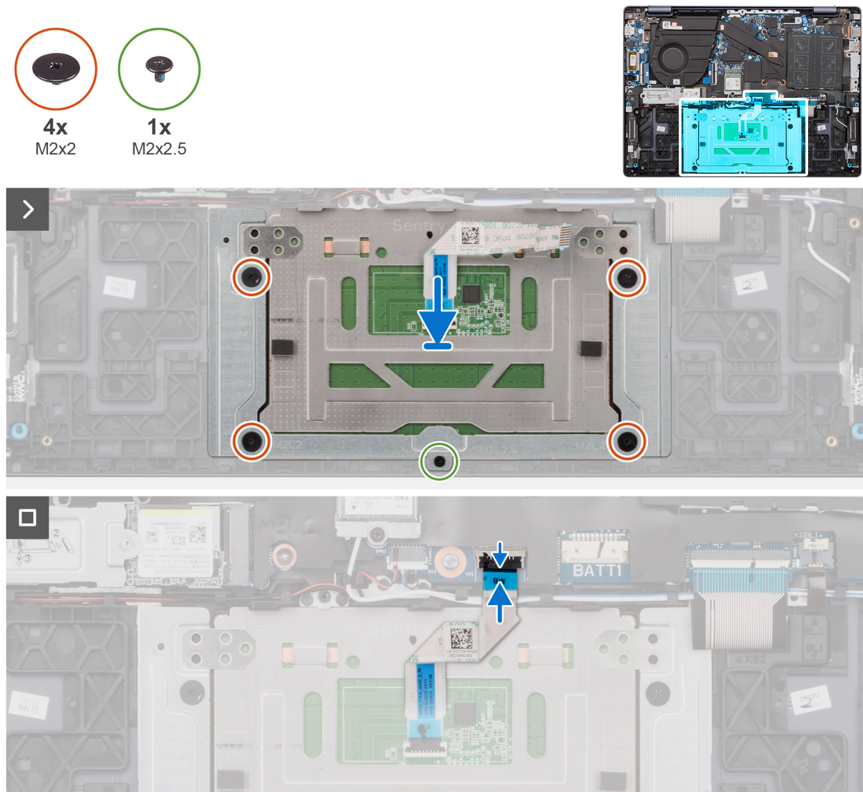
Rysunek 61. Instalowanie touchpada
