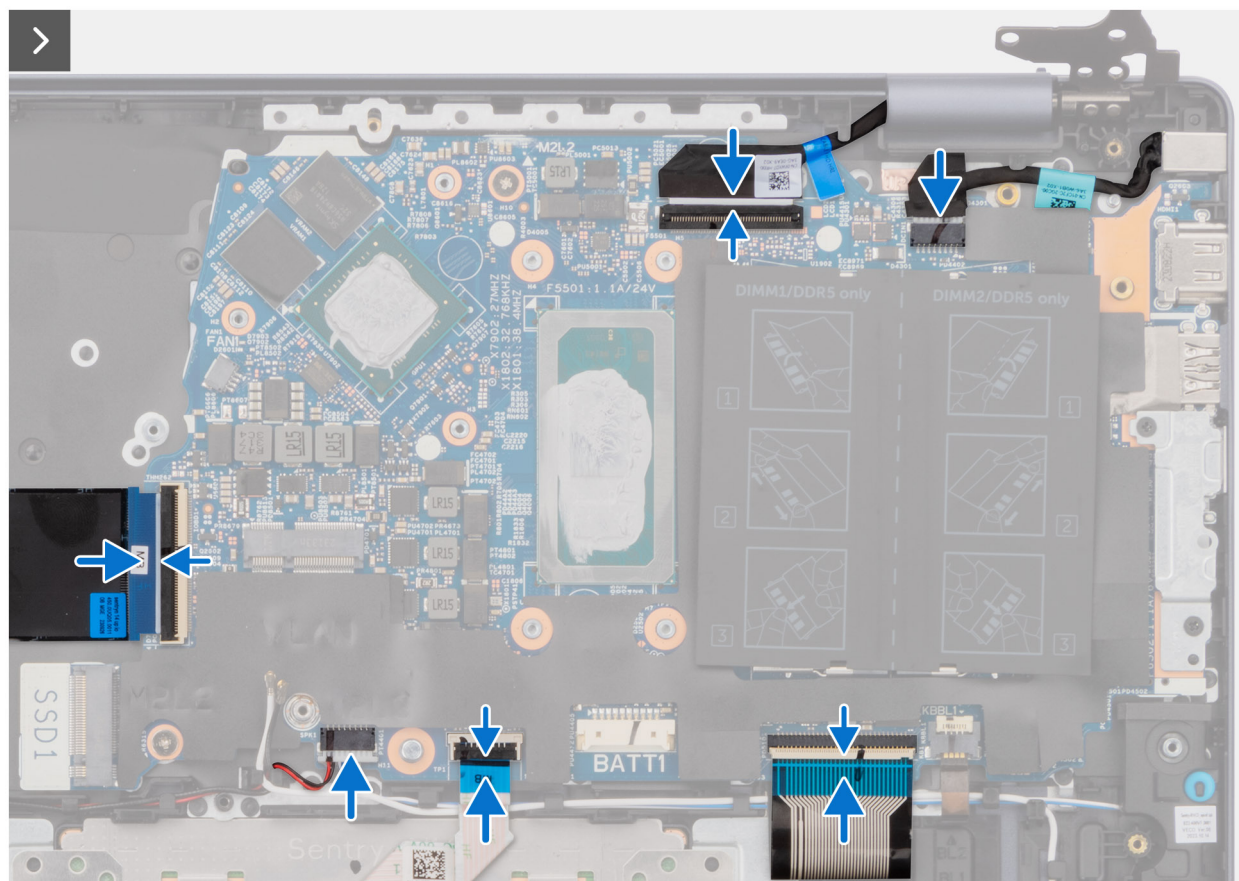
Rysunek 107. Instalowanie złączy kabli
