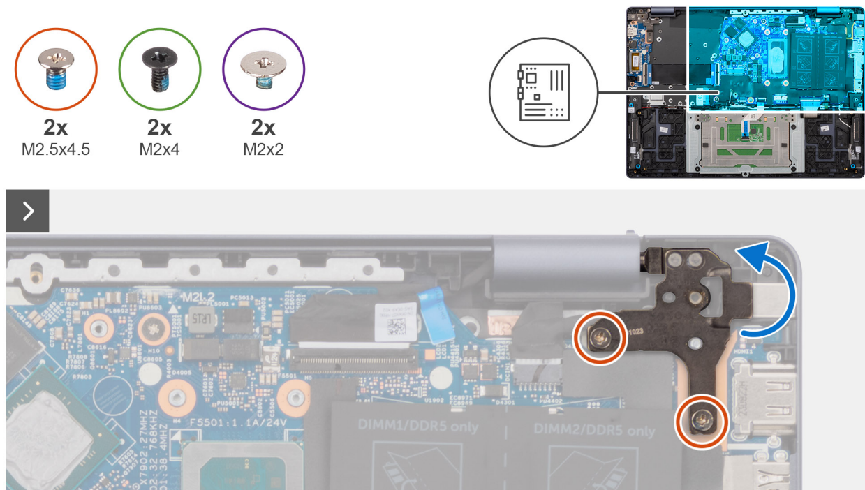
Rysunek 101. Wykręcanie śrub zawiasów
