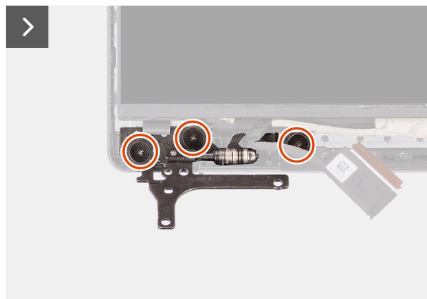
Rysunek 76. Wykręcanie śrub wyświetlacza
