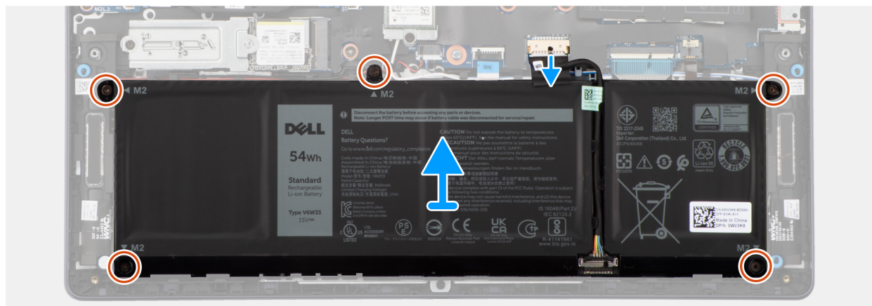
Rysunek 24. Wymontowywanie akumulatorów
