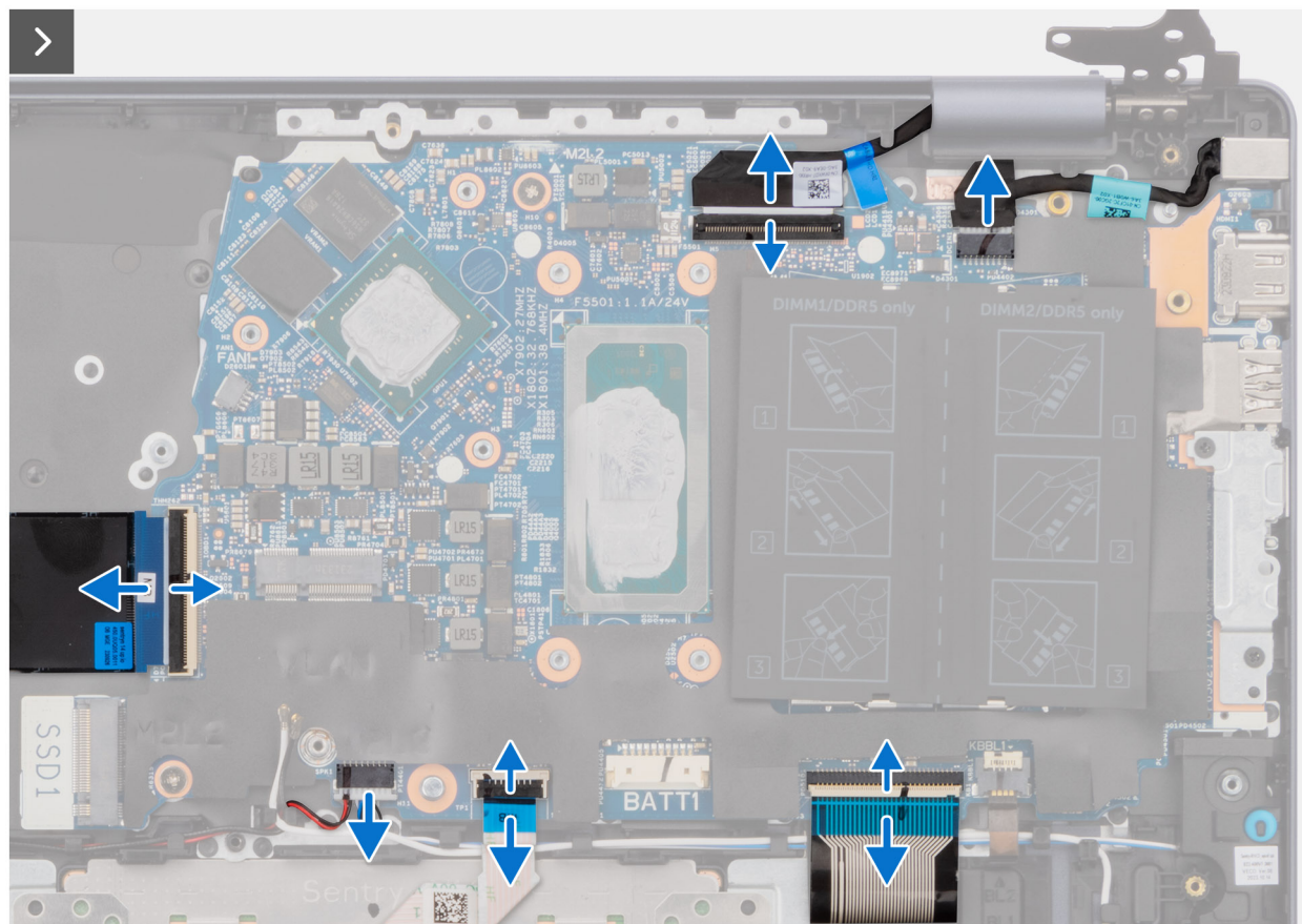
Rysunek 102. Wyjmowanie złączy kabli
