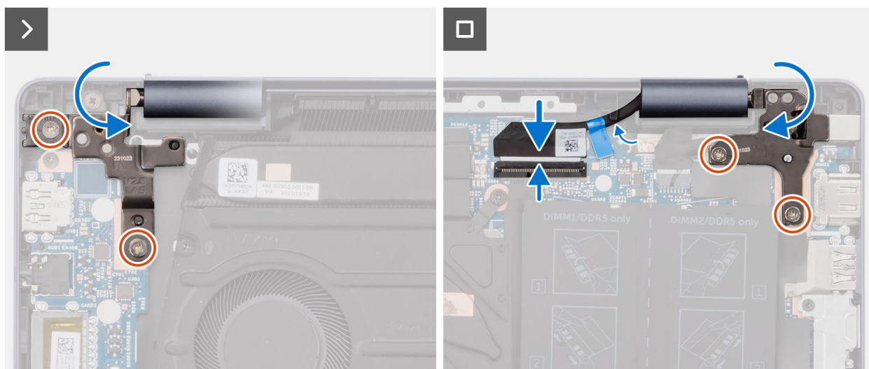
Rysunek 73. Wkręcanie
