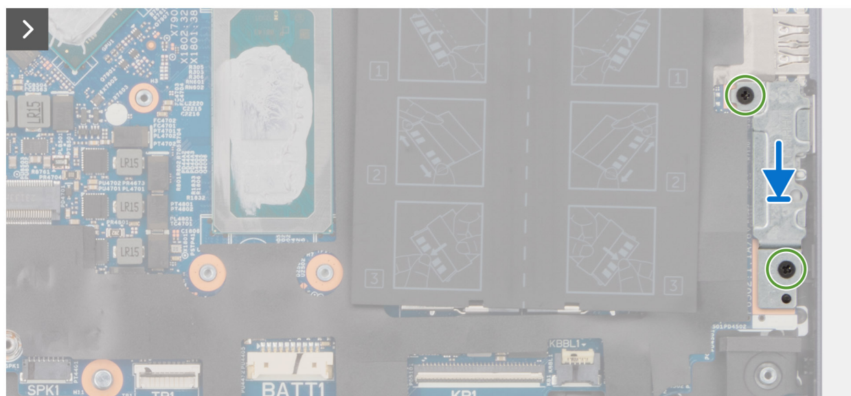
Rysunek 106. Instalowanie klamry portu USB Type-C
