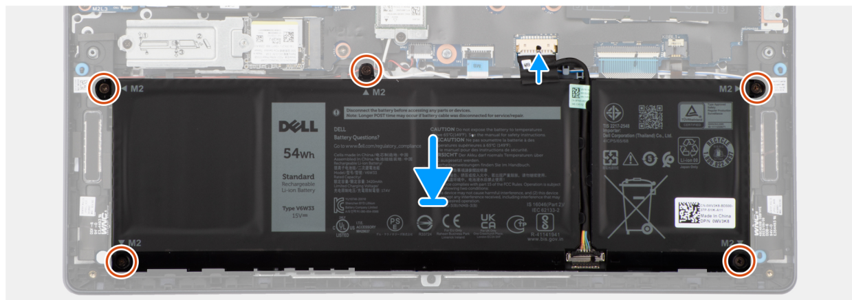
Rysunek 25. Instalowanie baterii
