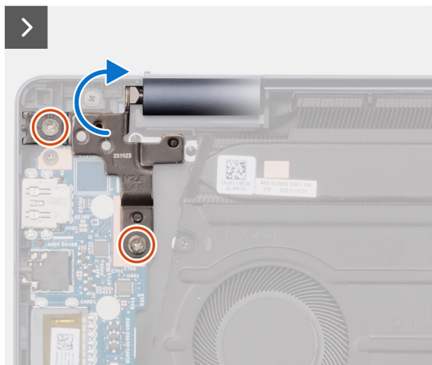
Rysunek 70. Wykręcanie śrub
