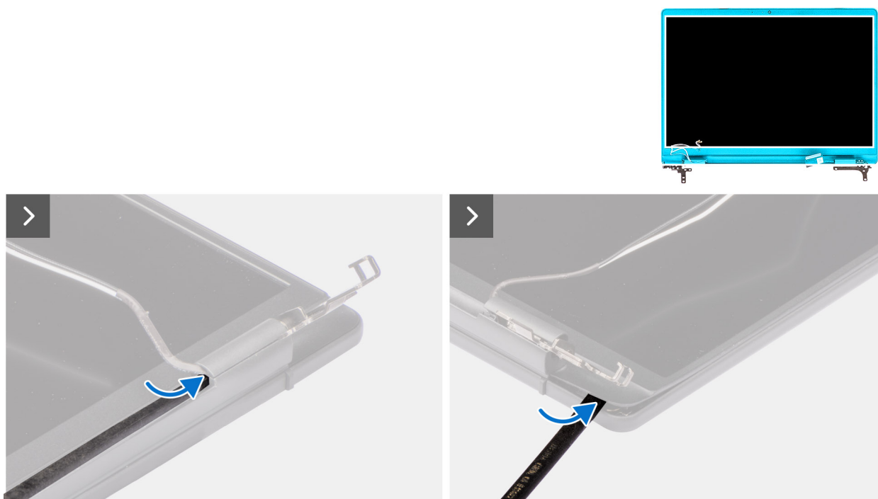
Rysunek 74. Wymontowywanie ramki wyświetlacza
