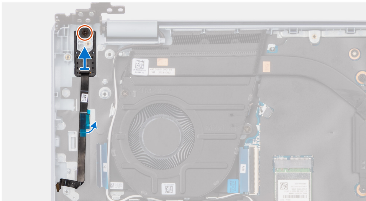
Rysunek 56. Wymontowywanie przycisku zasilania z czytnikiem linii papilarnych
