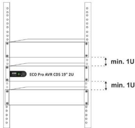
Rysunek 6: Montaż zasilacza w szafie
