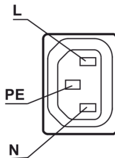
Rysunek 2: Układ wyprowadzeń gniazd wyjściowych SINLINE USB w wersji Rack
