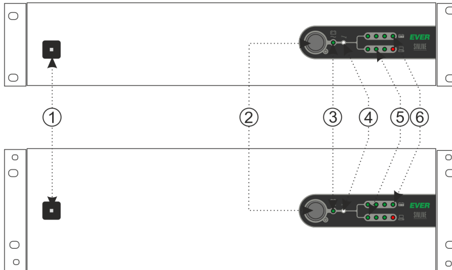
Rysunek 5: SINLINE USB 19" 2U i 3U - panel czołowy
