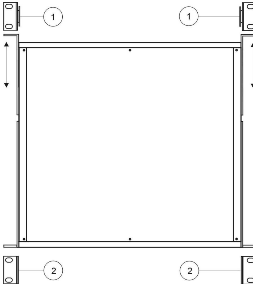
Rysunek 10: SINLINE USB 19" - widok zasilacza z góry
