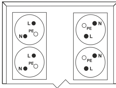
Rysunek 14: Układ wyprowadzeń gniazd wyjściowych SINLINE USB w wersji Tower
