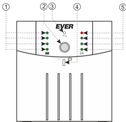
Rysunek 1: SINLINE USB HID wersja Tower - panel czołowy
