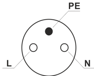
Rysunek 11: Układ wyprowadzeń gniazda zasilającego
