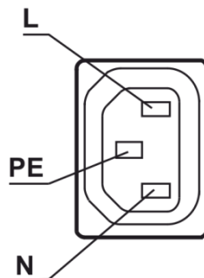
Rysunek 15: Układ wyprowadzeń gniazd wyjściowych SINLINE USB HID w wersji Rack
