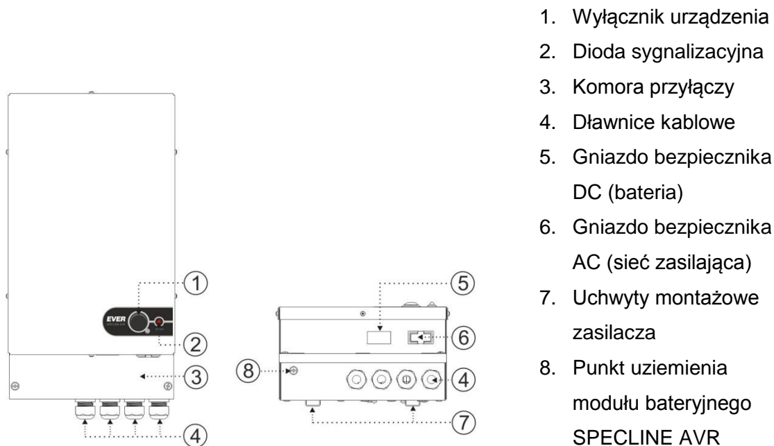
Rysunek 1: Widok panelu przedniego zasilacza SPECLINE AVR Pro 700
