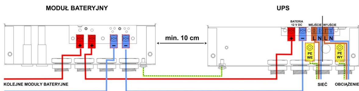
Rysunek 8: Podłączenie modułu bateryjnego
