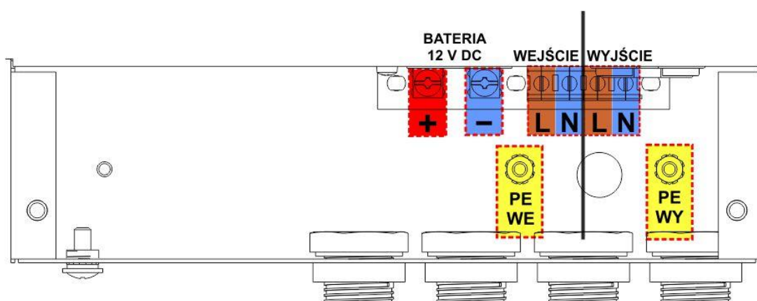
Rysunek 4: Elementy przyłączeniowe zasilacza
