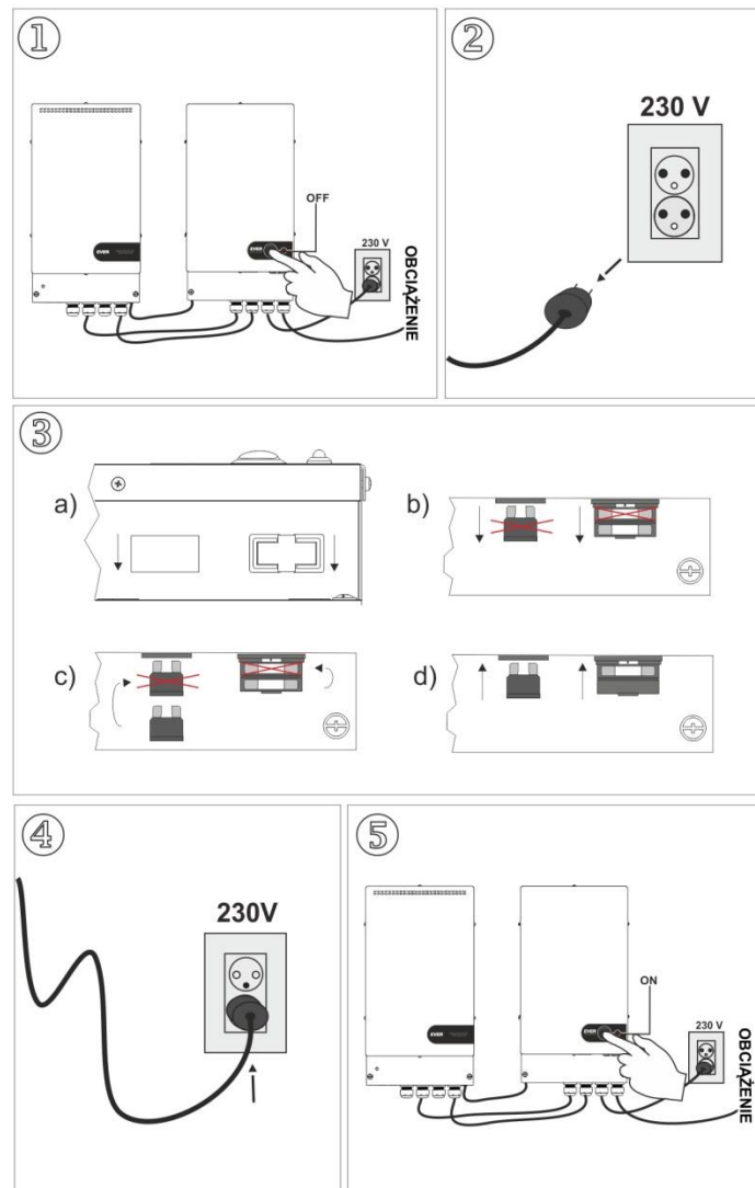
Rysunek 9: Wymiana bezpieczników
